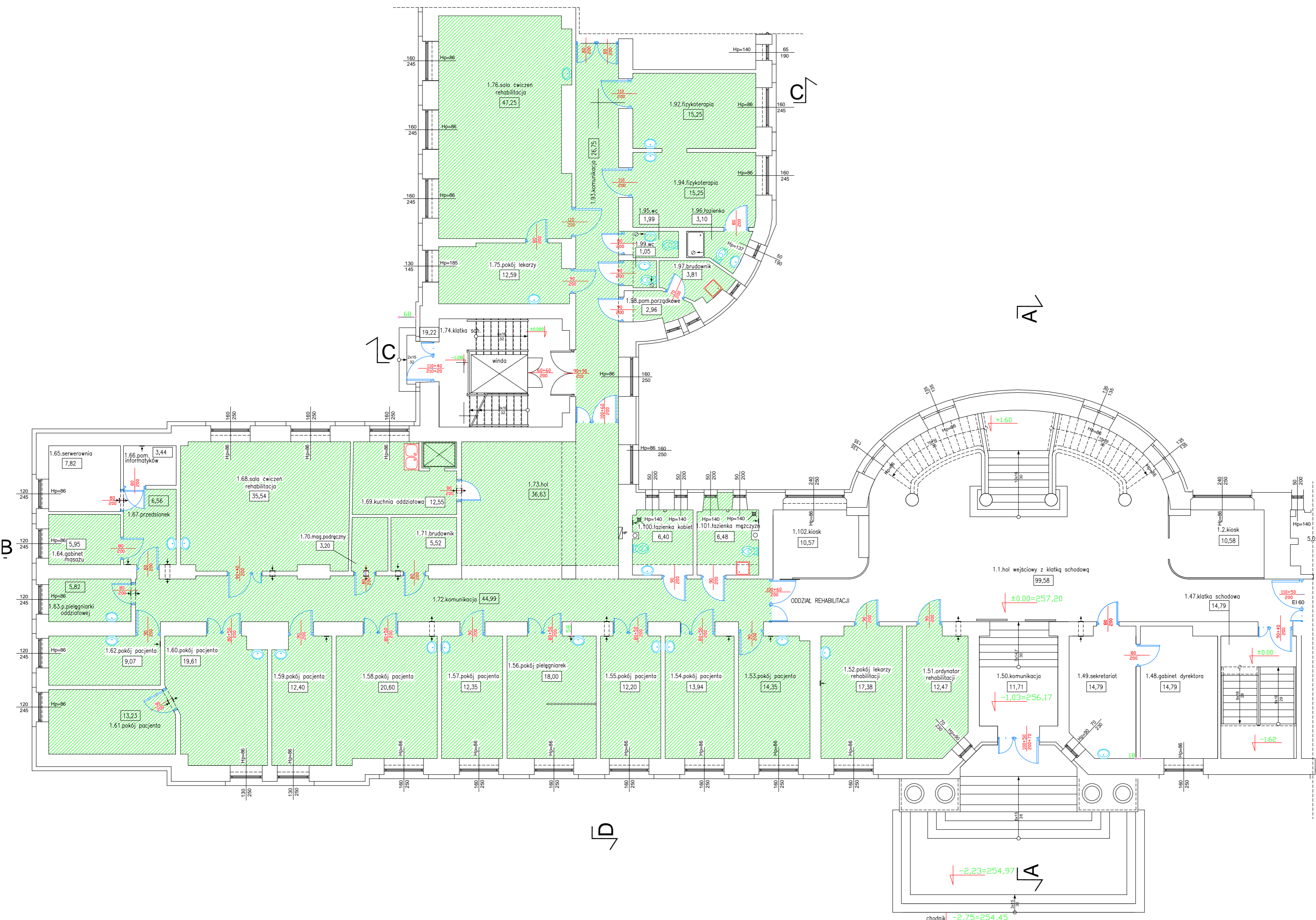
Rzut parteru skala 1:100 ODDZIAŁ REHABILITACJI
